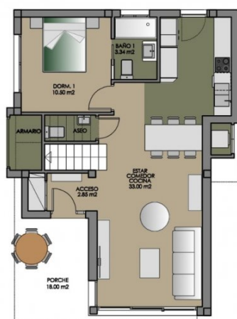
PLANTA BAJA
