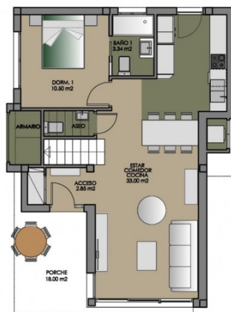
PLANTA BAJA
