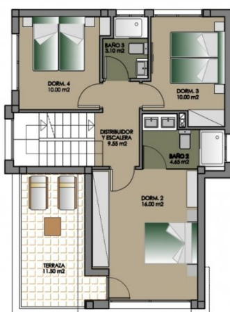
PLANTA PISO
