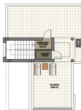
CUBIERTA
