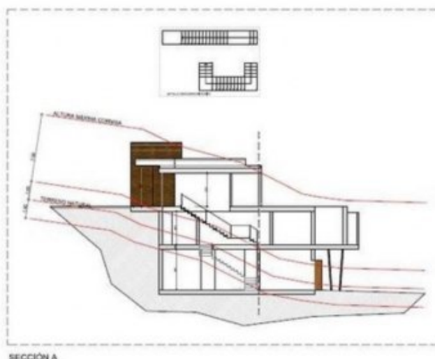
SECCIÓN A
